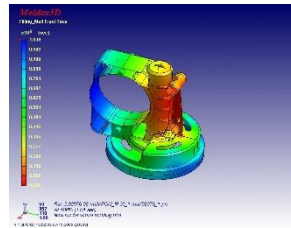
模流分析 Moldflow Analysis
