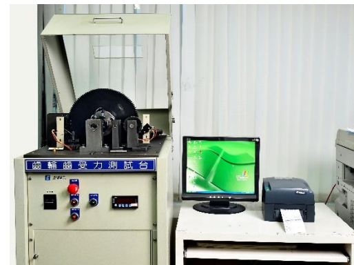
齒輪強度測試機 Gear Torque Tester
